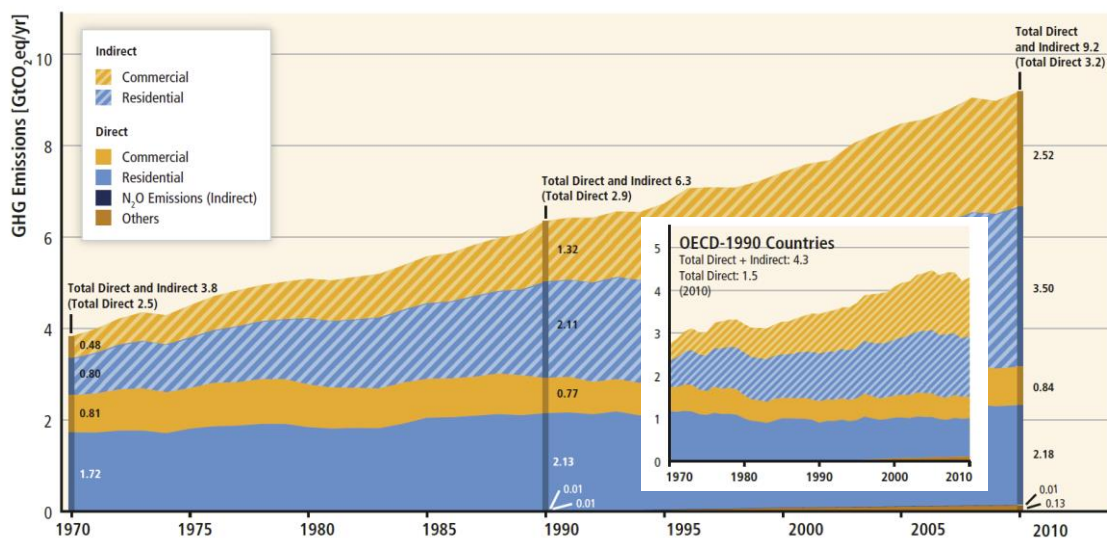
Figur 1: Energi til bygg – relaterte klimagassutslipp globalt og for OECD land (innfelt) (IPCC, ar5, wg3)
